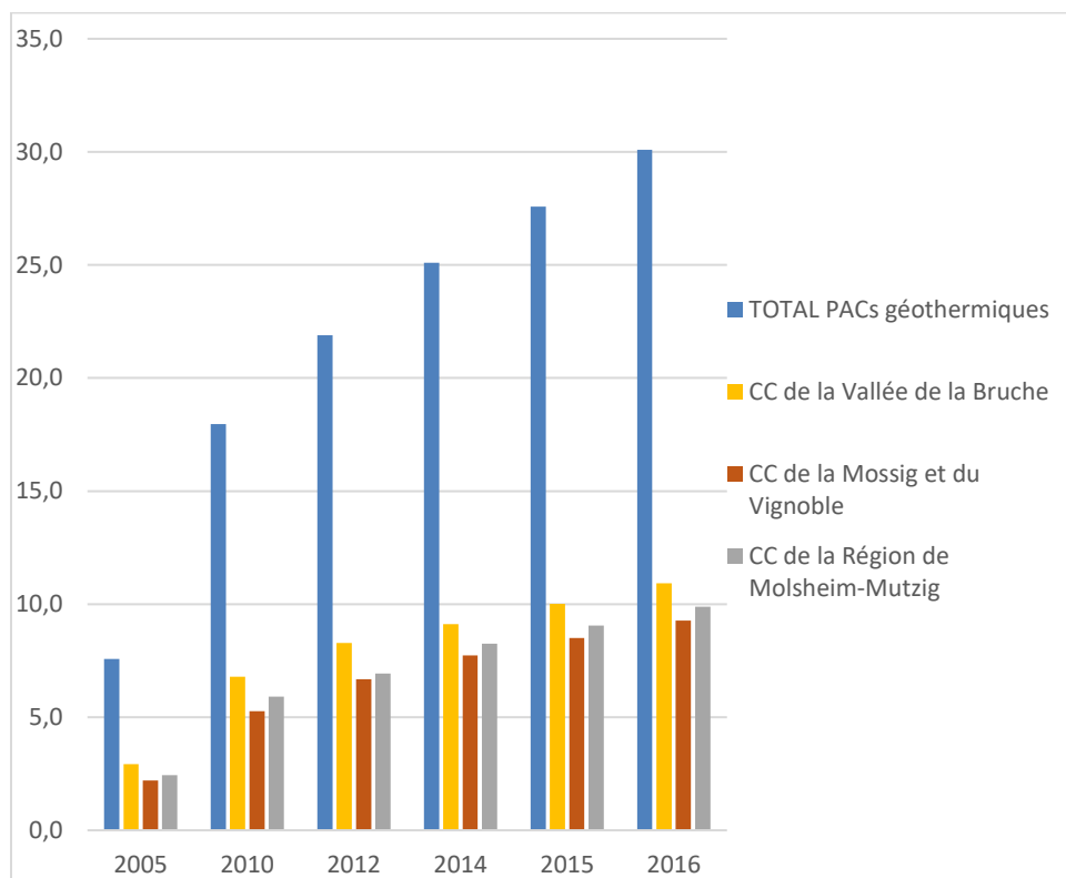
Graphique n°29. Evolution de la production des PACs géothermiques en GWH/an par EPCI
