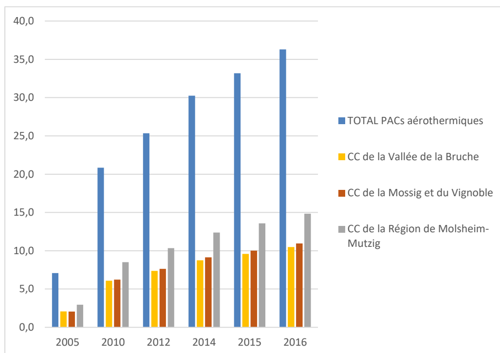
Graphique n°28. Evolution de la production des PACs aérothermiques en GWH/an par EPCI
