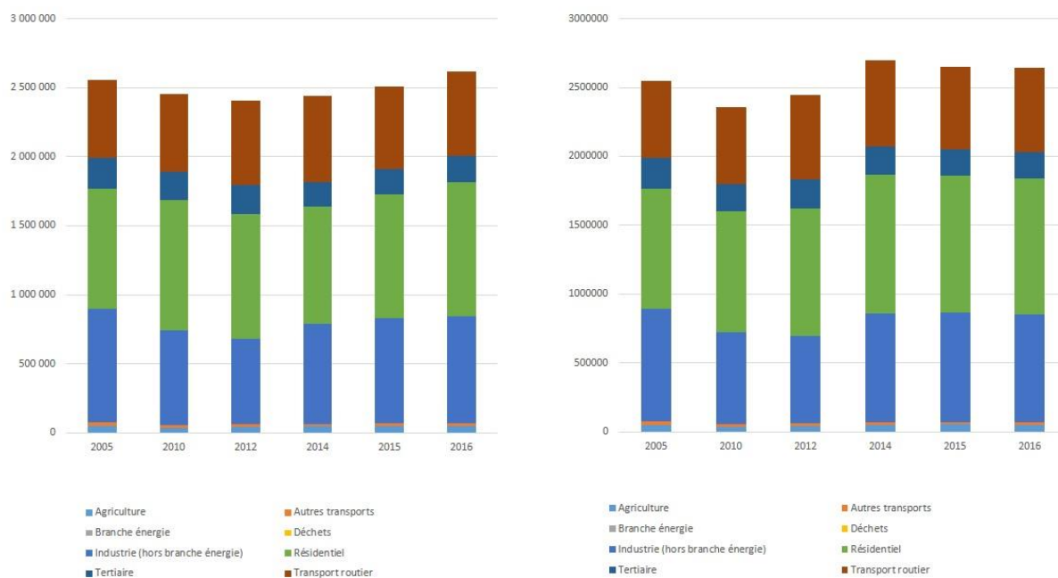
Graphique n°5. Consommations énergétiques finales entre 2005 et 2016 pour le territoire Bruche Mossig (à gauche non corrigée du climat, et à droite corrigée du climat)
