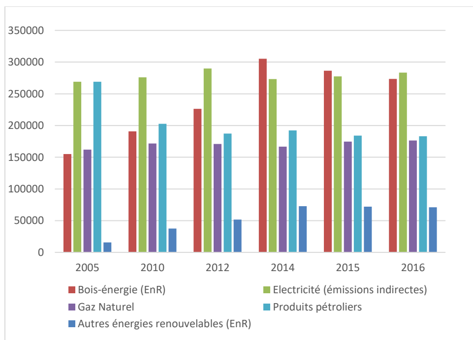
Graphique n°9. Evolution de la consommation énergétique entre 2005 et 2016 pour le territoire Bruche-Mossig pour le secteur résidentiel par source d'Énergie en MWh
