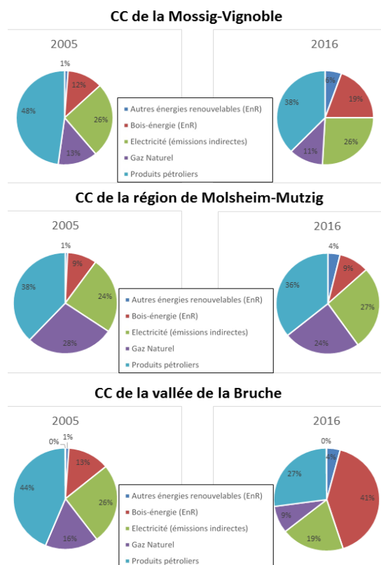
Graphique n°59. Consommation énergétique finale corrigée des variations climatiques par source d'énergie sur les différentes communautés de communes
