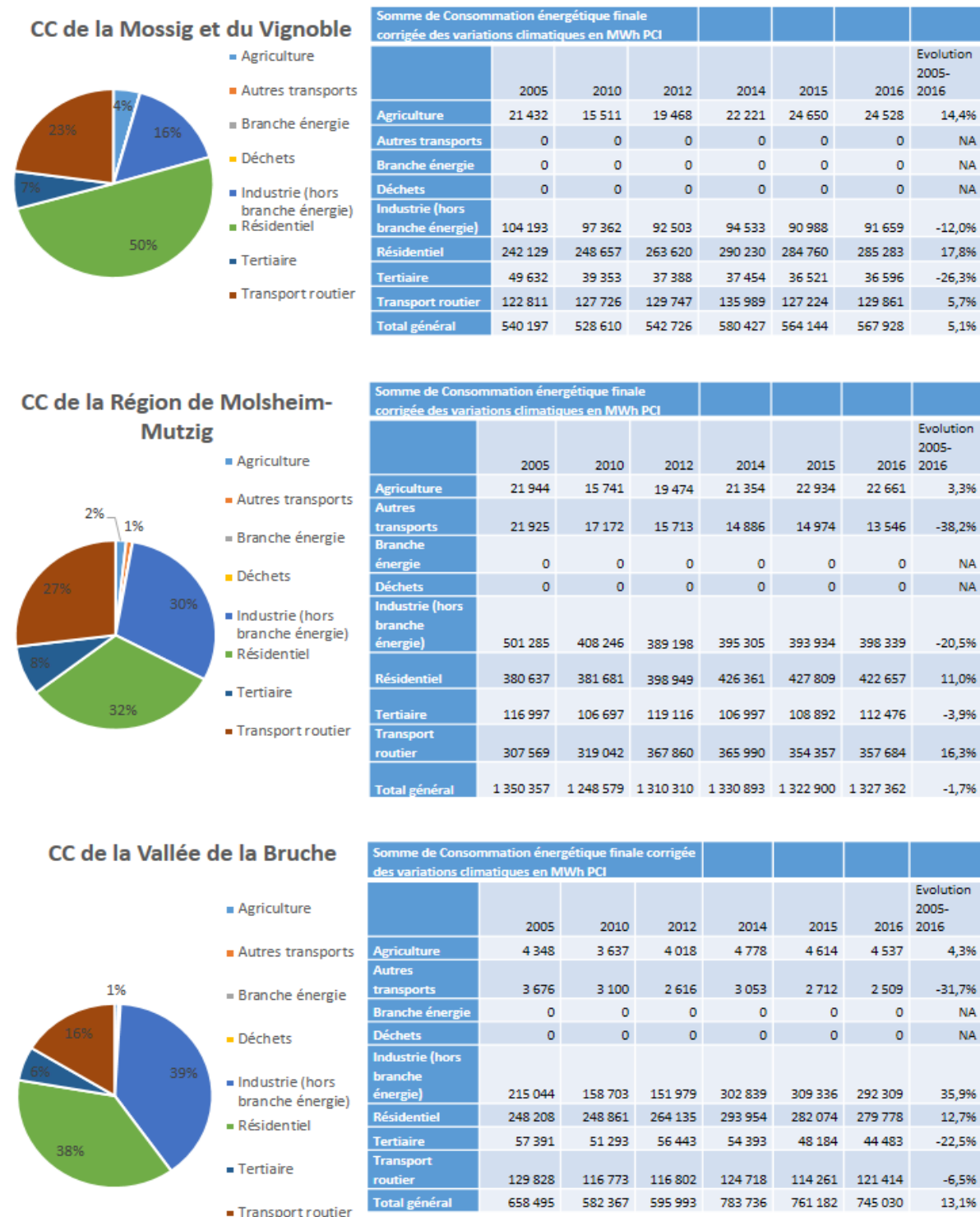
Graphique n°6. Portrait type des consommations énergétiques (corrigées du clim at) en MWh des 3 Communautés de communes du territoire de 2005 à 2016
