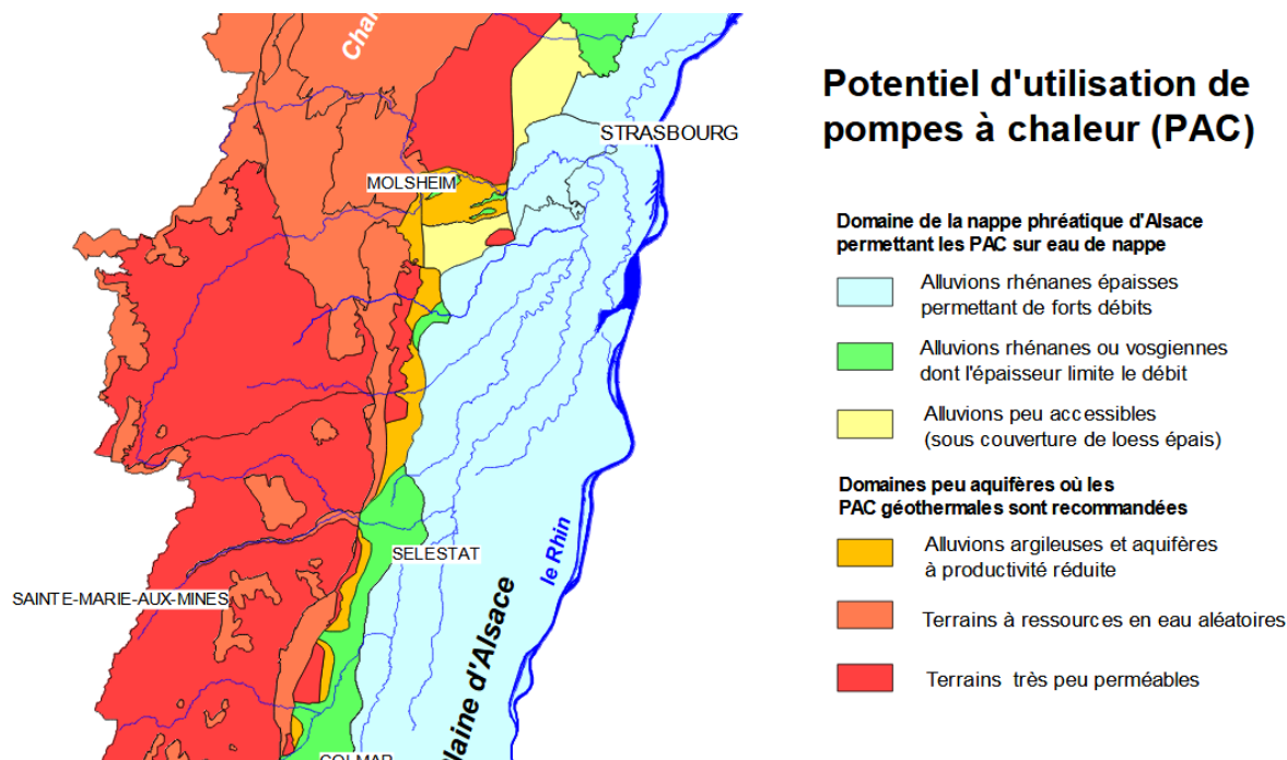
Carte n°10. Le potentiel d'utilisation pour les pompes à chaleurs
