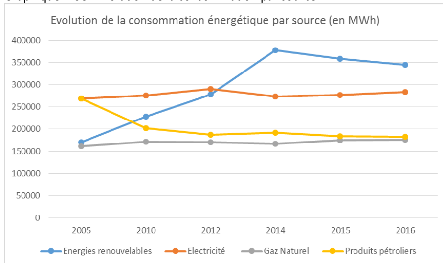
Graphique n°58. Evolution de la consommation par source
