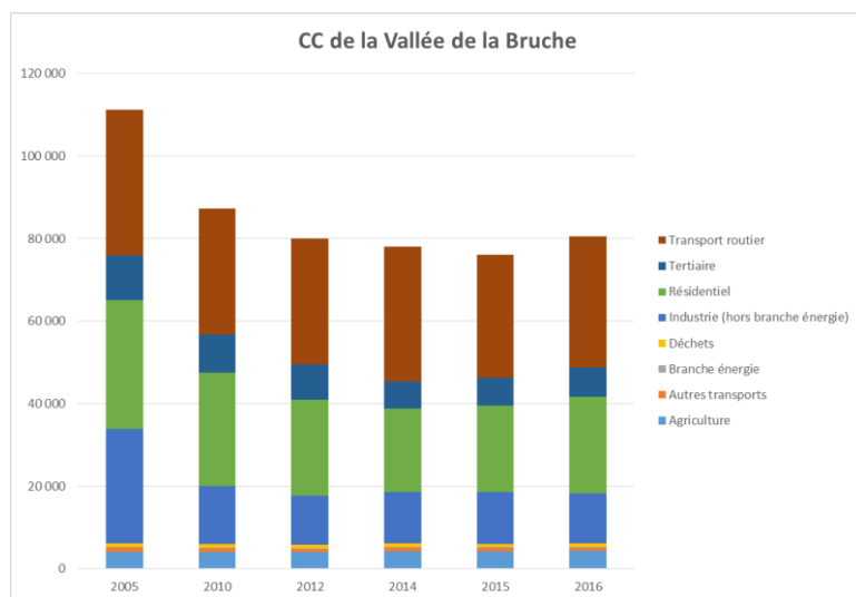
Graphique n°41. Evolution des émissions en équivalent en tonnes-équivalent de CO2 par secteur entre 2005 et 2016 sur la CC de la vallée de la Bruche
