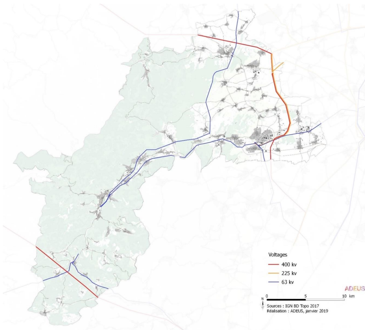
Carte n°13. Les lignes électriques sur le territoire Bruche-Mossig
